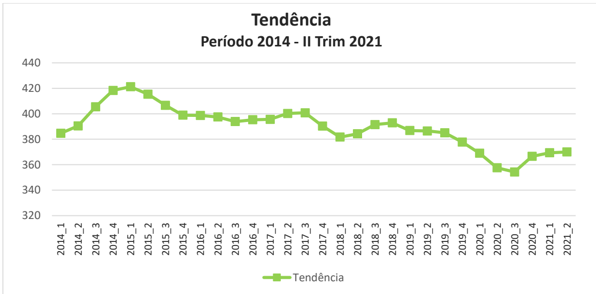
Gráfico 6 – PIB_Tendência
