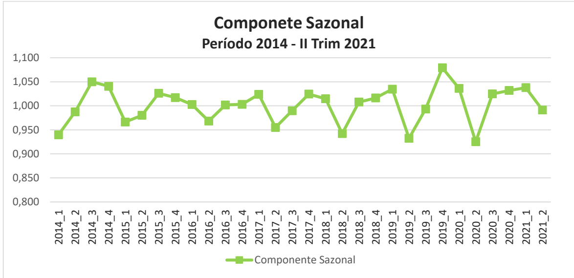
Gráfico 7 – PIB_Componente Sazonal
